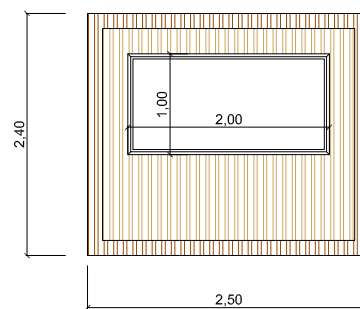
ALZADOS
