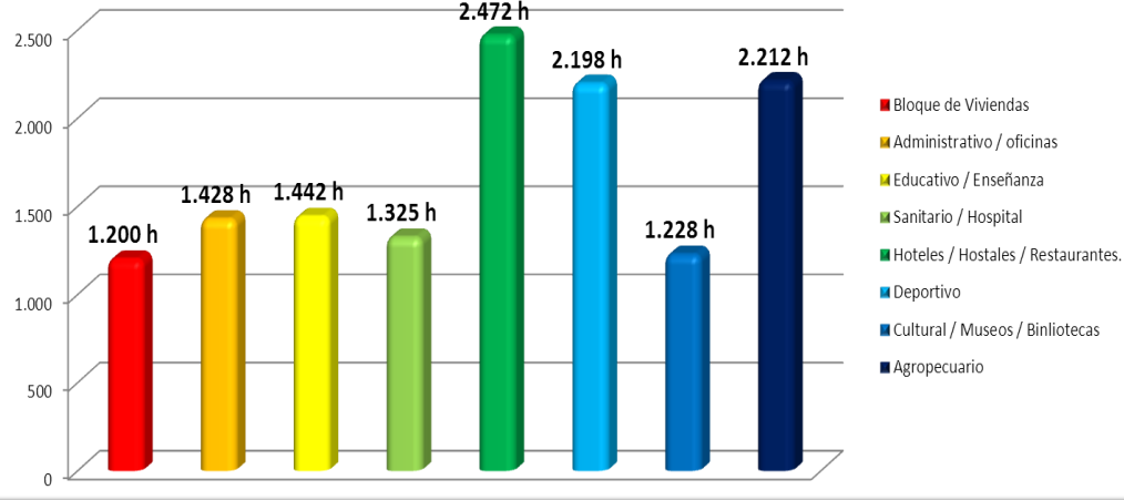
Media de horas equivalentes por tipo de edificio
