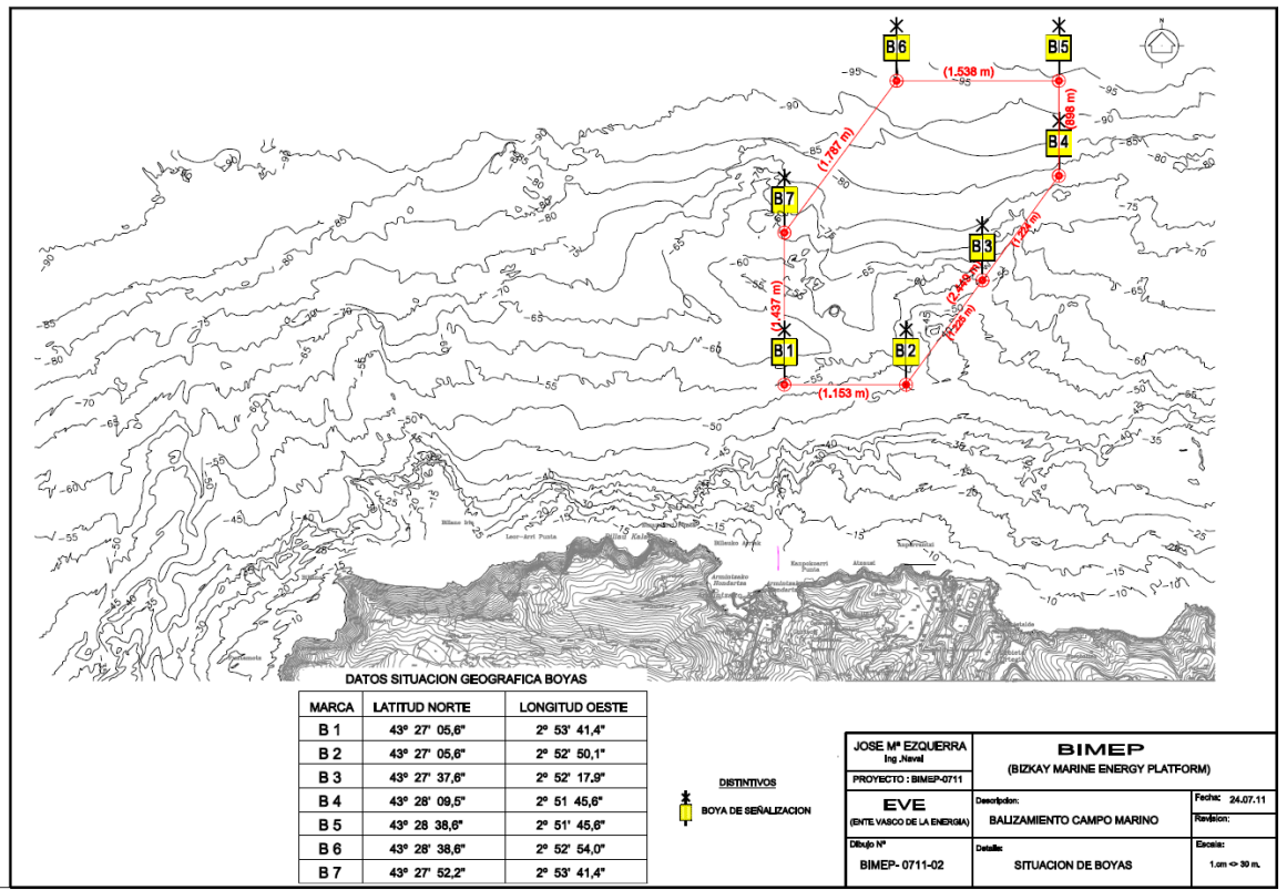
Figura 1 Disposición de las boyas de balizamiento
