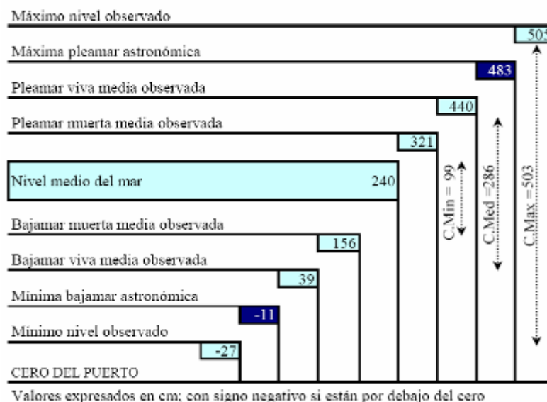
Figura 4. Carrera de marea del mareógrafo del puerto de Bilbao
